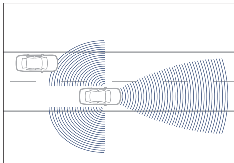
Lane Keeping Assist registrerer kantlinjene i veibanen og varsler føreren dersom bilen beveger seg ut av veien uten bruk av blinklys. Dødvinkelassistenten kontrollerer dødvinkelen og varsler når et annet kjøretøy befinner seg i den.
